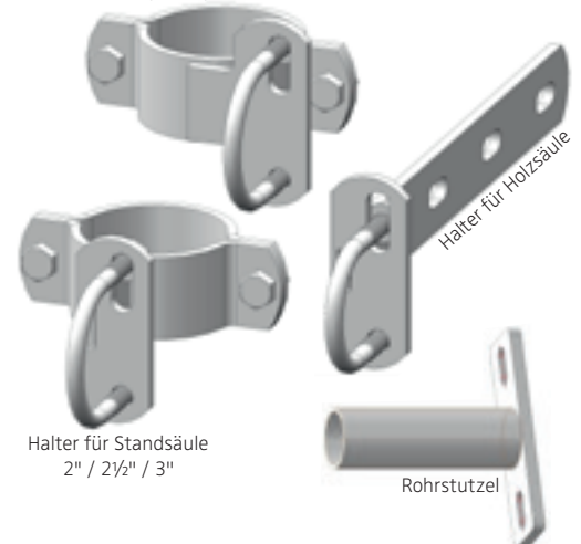
Halter für Standsäule 0cm Abstand 2" / 2½" / 3"
