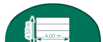
Giebel für Sektionaltor Torbreite 4 m; Höhe variabel
