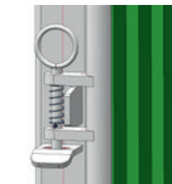
Federverschluss mit einstellbarer Türe
