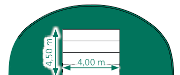
Giebel für Sektionaltor Torbreite 4 m; Höhe variabel
